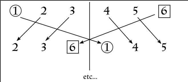
Kreuzspiel permutation pattern
